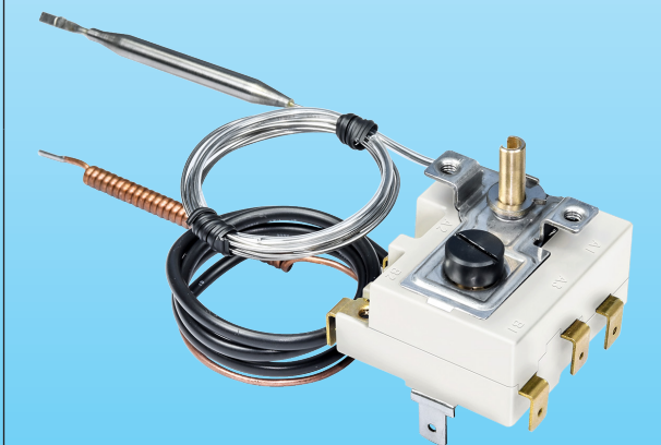
Pulsante di reset protetto da tappo M10
